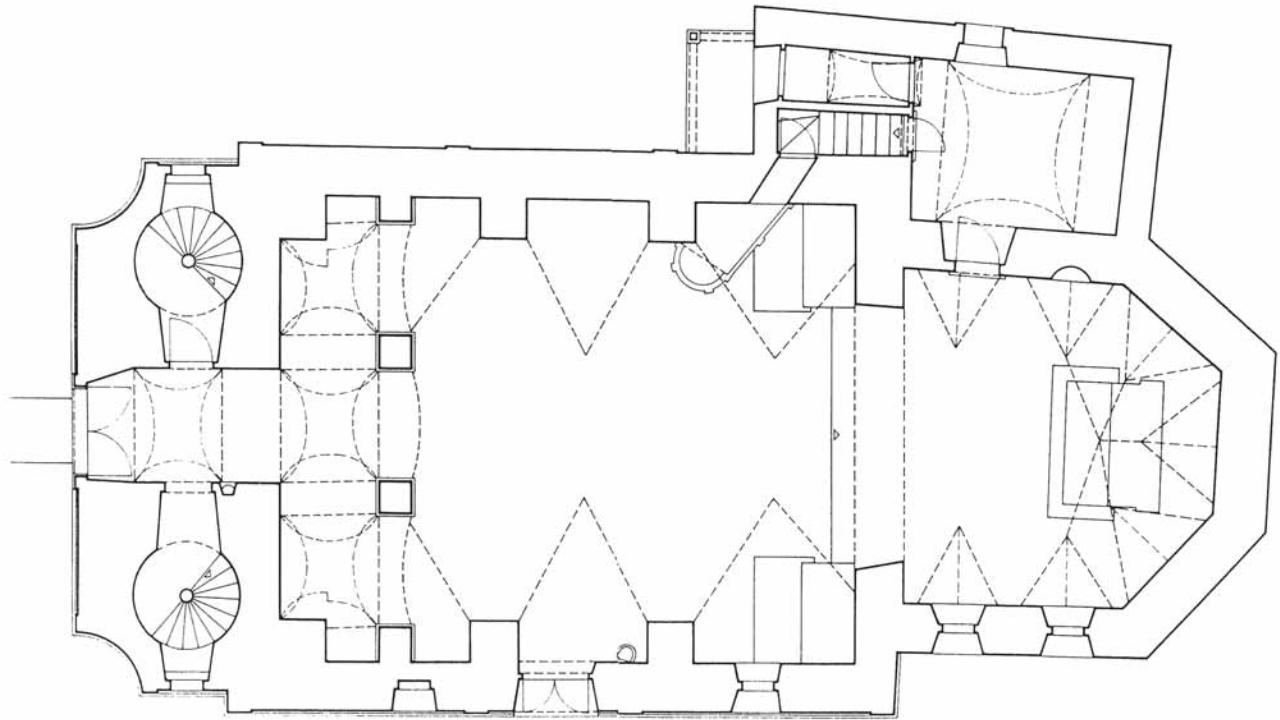
1. Velika Erpenja, župna crkva sv. Tri kralja, tlocrt, planoteka Instituta za povijest umjetnosti
