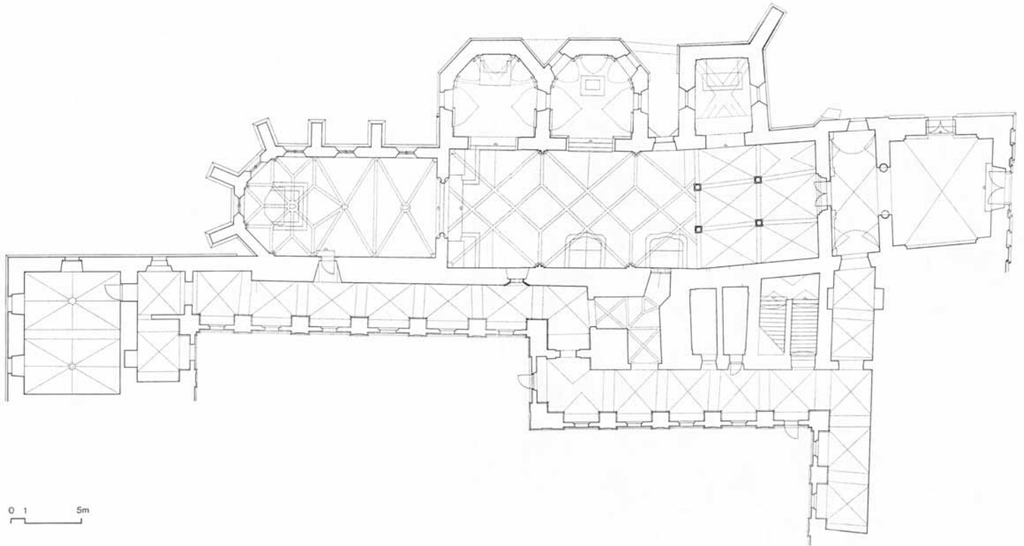
8. Lepoglava, pavlinski samostan i crkva sv. Marije, tloert, planoteka Instituta za povijest umjetnosti
