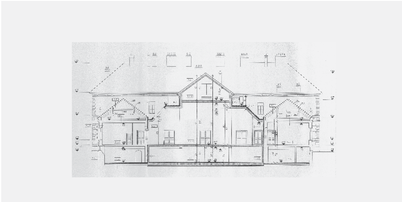
Presjek (C–C) s pogledom na sjever
