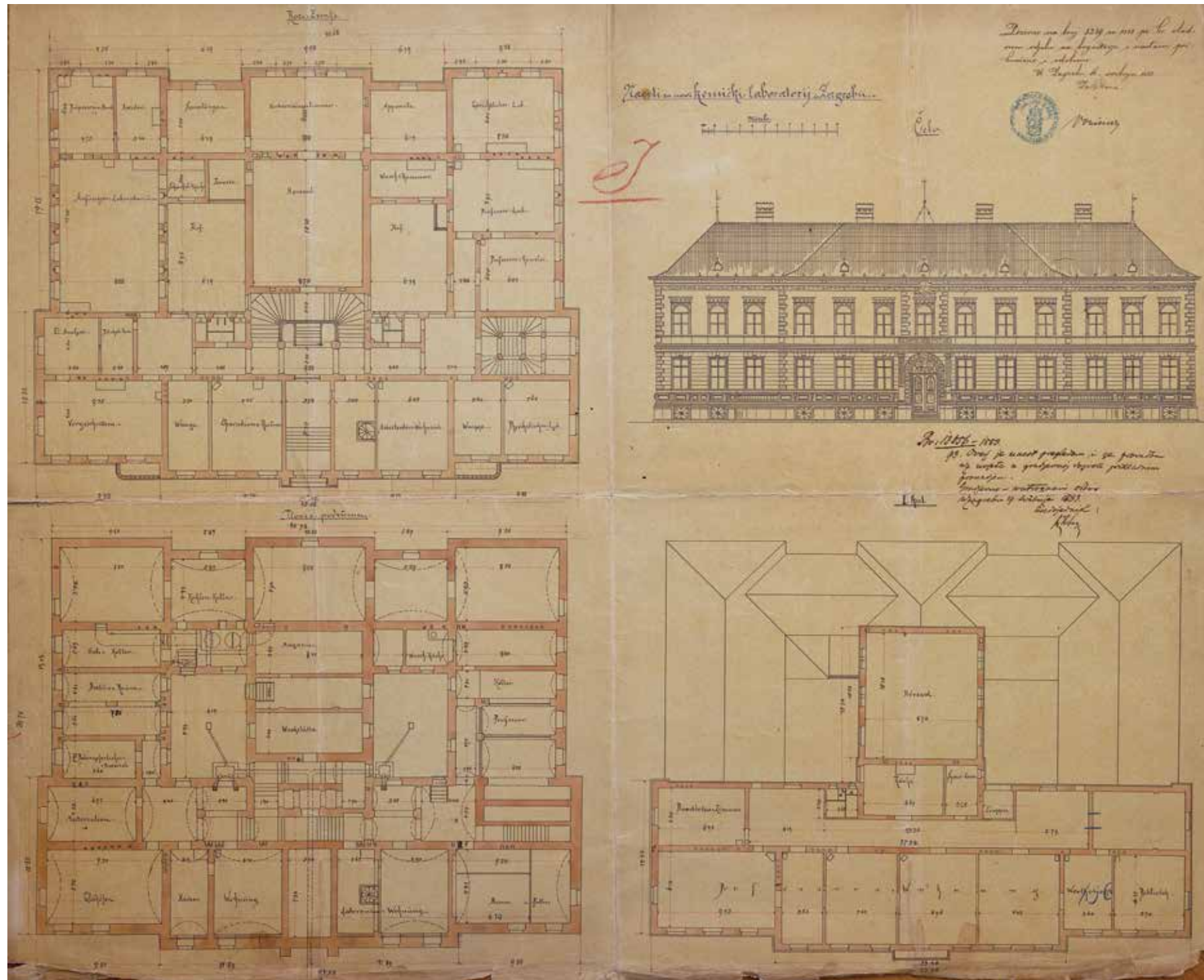
Herman Bollé, Kemijski laboratorij, tlocrti podruma, prizemlja, prvog kata i sjeverno pročelje, projekt одобren 29. svibnja 1883., HDA
