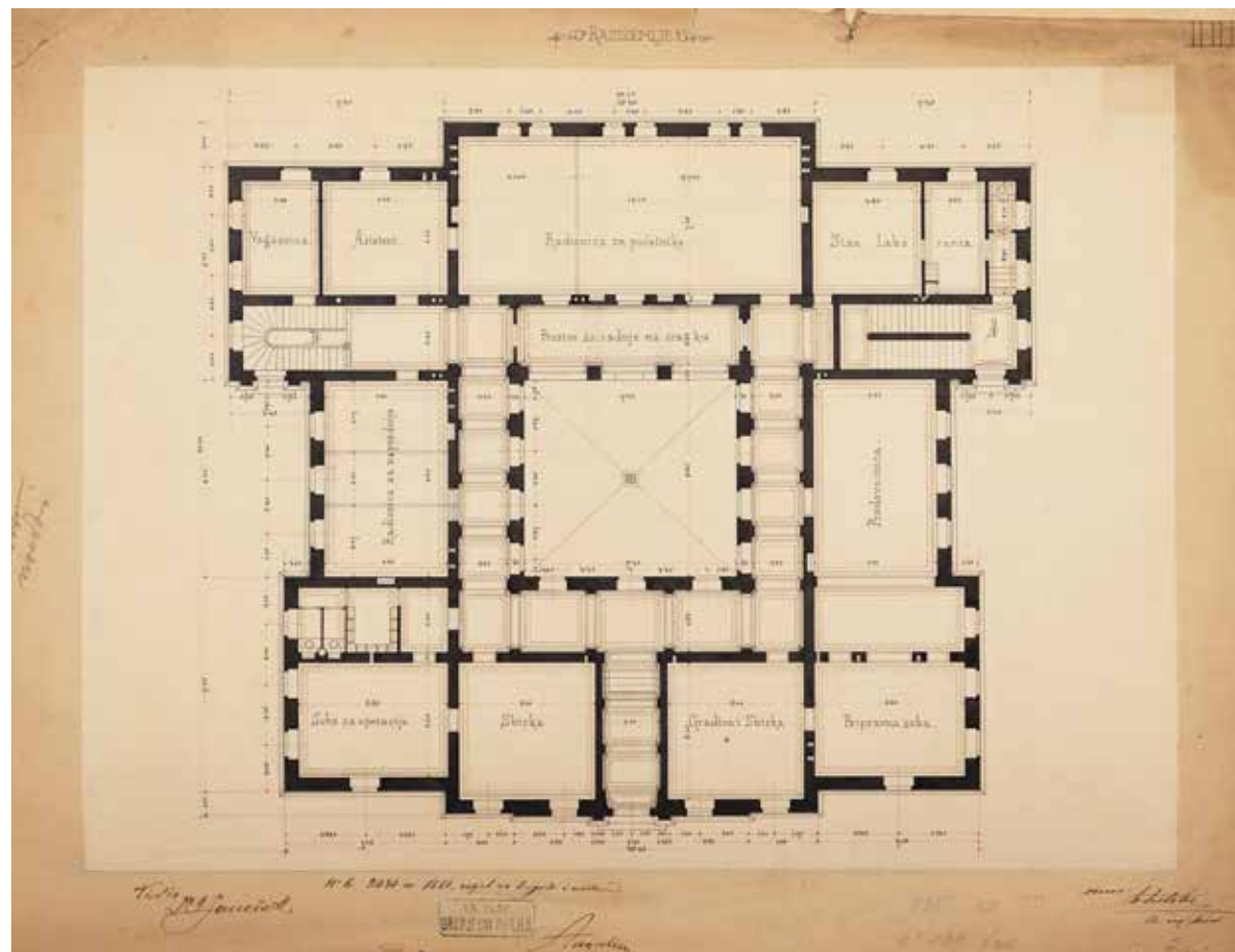
Matija Antolec, Kemijski laboratorij, tlocrta podruma, prizemlja, prvog kata i presjek (varijanta s jednokatnom zgradom), 1881., HDA
